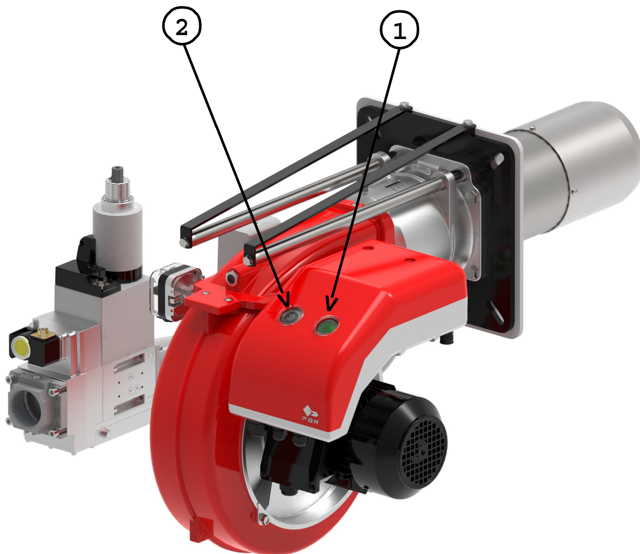
Fig. 4 Segnalazioni bruciatore
