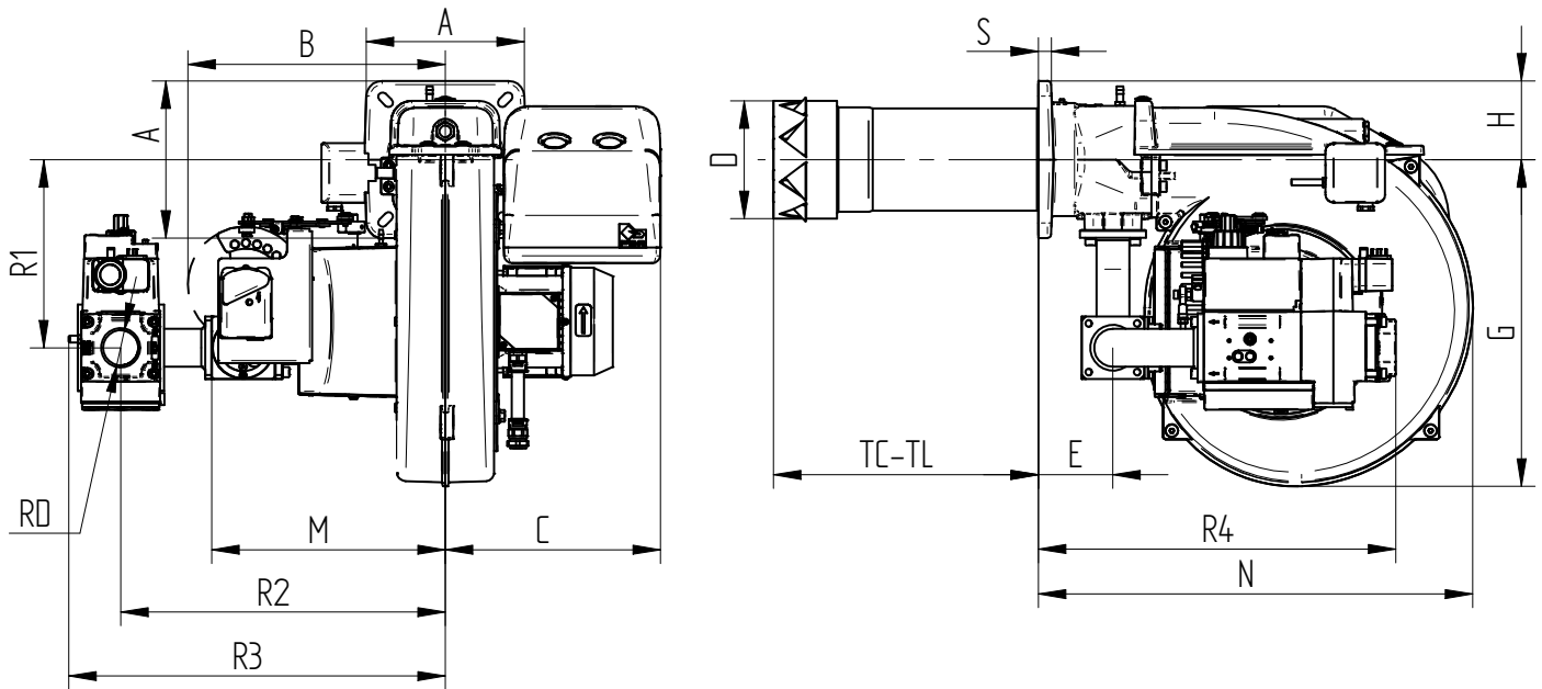
Fig. 3 Dimensioni ingombro GAS XP60/MCE-LX-EVO
