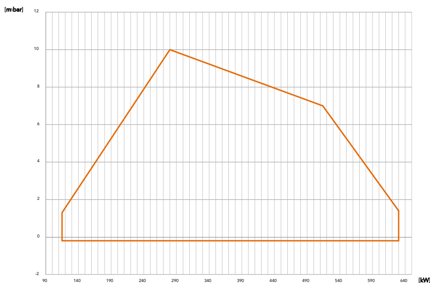
Fig. 2 X = Potenza termica Y = Pressione in camera di combustione
